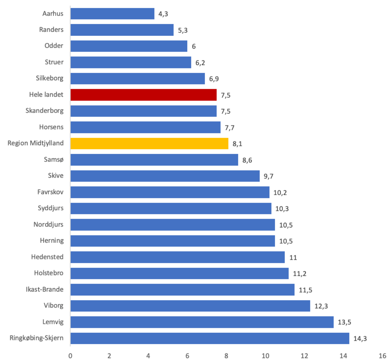
Figur 3. CO2-udledning per indbygger, ton, 2018
